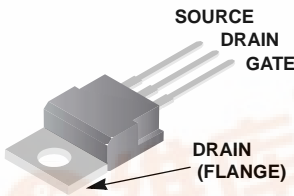
JEDEC TO-220AB
