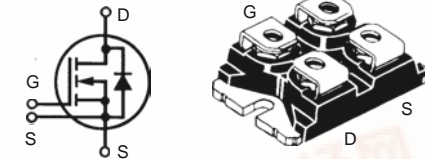
miniBLOC, SOT-227 B (IXFN) E153432
