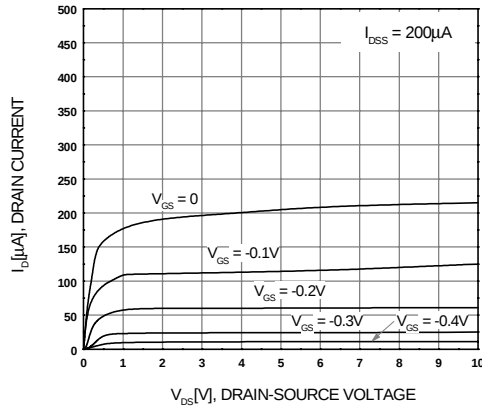
Figure 1. I_D - V_{DS}
