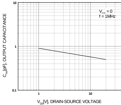
Figure 7. C_{RSS} - V_{DS}
