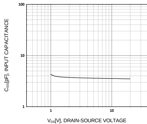
Figure 6. C_{iss} - V_{DS}
