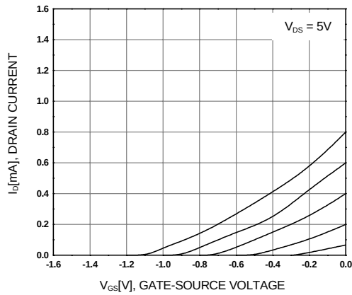
Figure 3. I_D - V_{GS}
