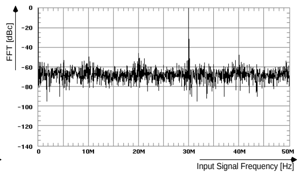
Spectrum @30MHz 1)
