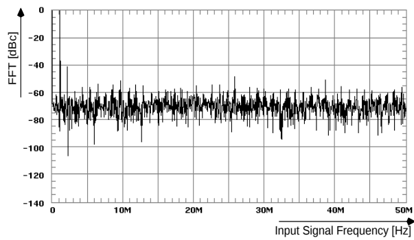
Spectrum @1MHz 1)
