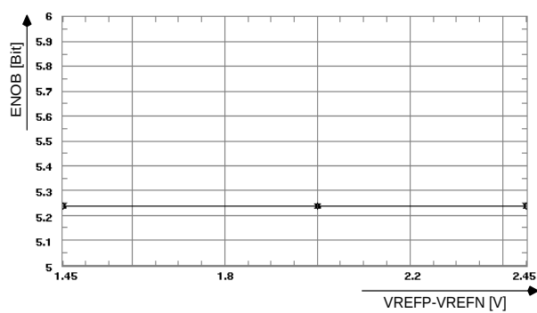
ENOB vs ( V_{\text{REFP}}-V_{\text{REFN}} ) @30MHz
