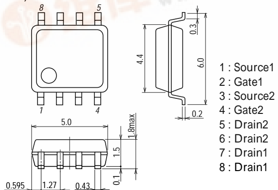
外形図 2129 (unit : mm)
