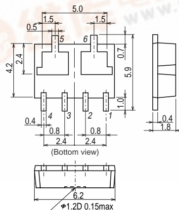
外形図 2118 (unit : mm)
