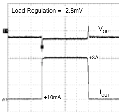
I_{OUT} = +10mA \rightarrow +3A \rightarrow +10mA
