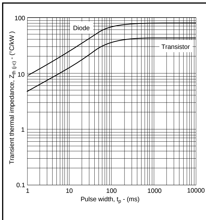
Fig. 12 Transient thermal impedance
