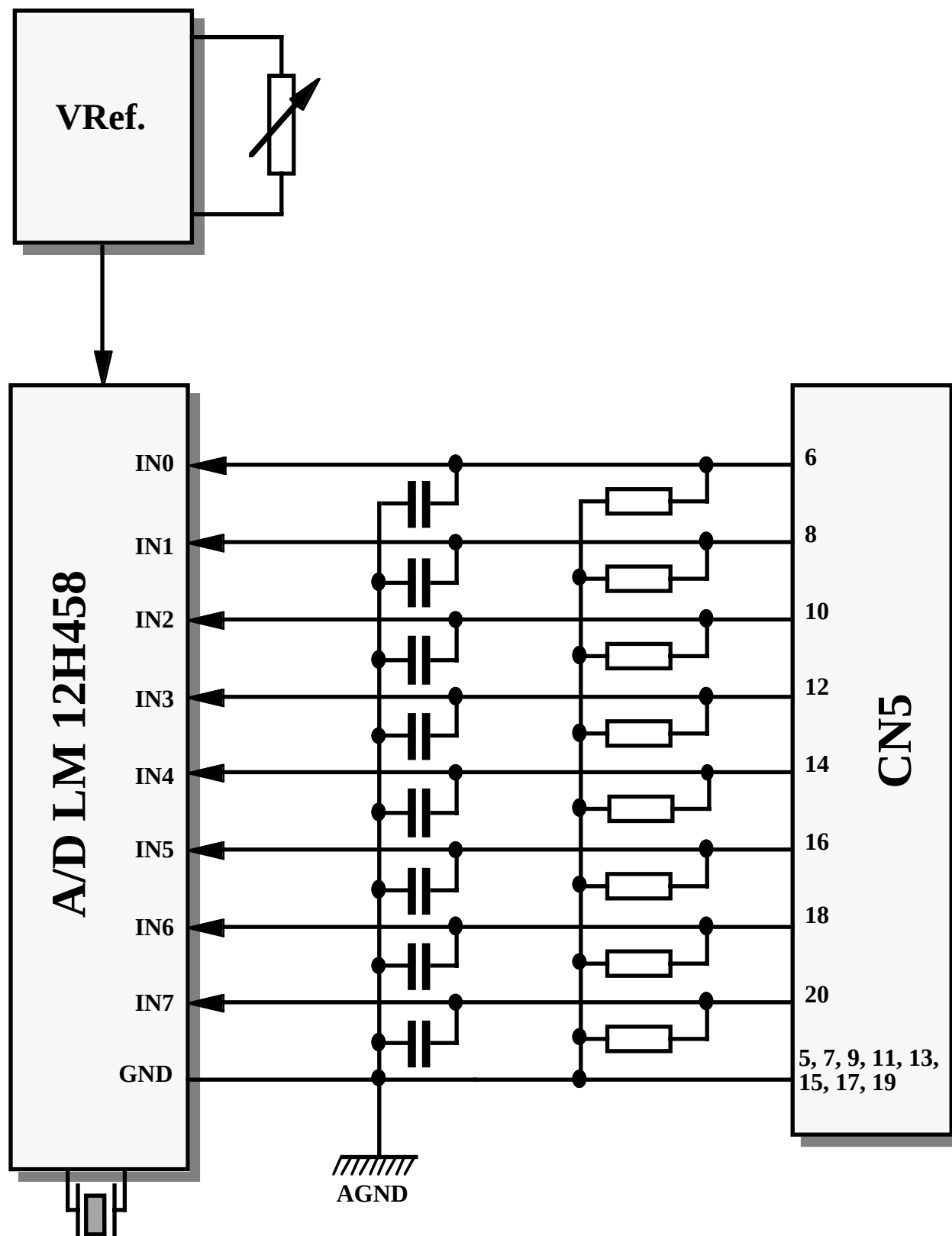
FIGURA 7: SCHEMA D'INGRESSO A/D CONVERTER
