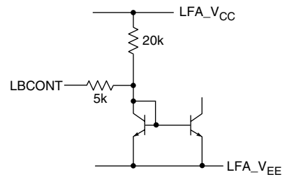
Fig. 11 LBCONT Circuit
