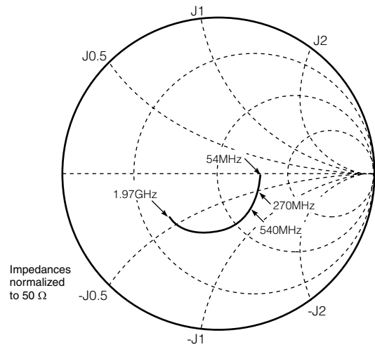
Fig. 15 Input Impedance
