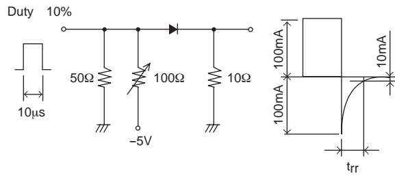
t_{rr} 指定回路図 (SBD部)
