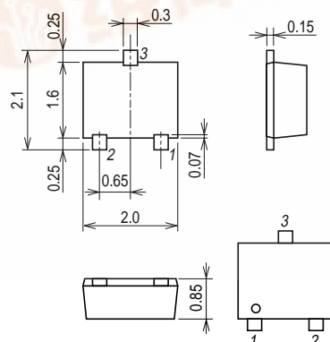
外形図 2167A
