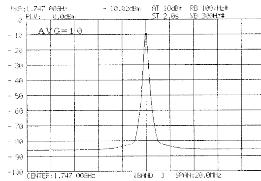
b-2. Spectrum2(1747MHz,PN9)
