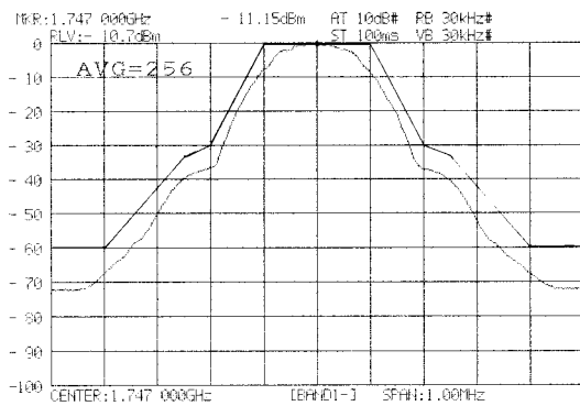
b-1. Spectrum1(1747MHz,PN9)
