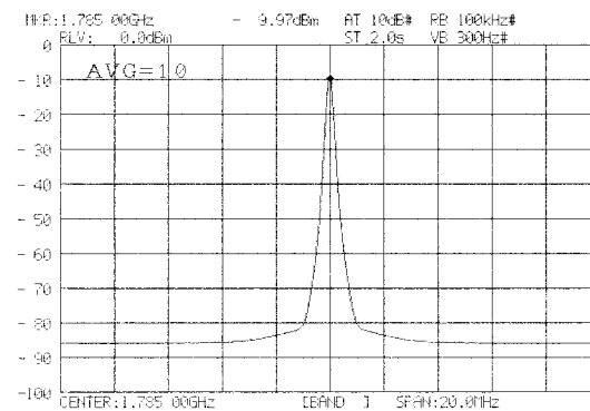
c-2. Spectrum2(1785MHz,PN9)
