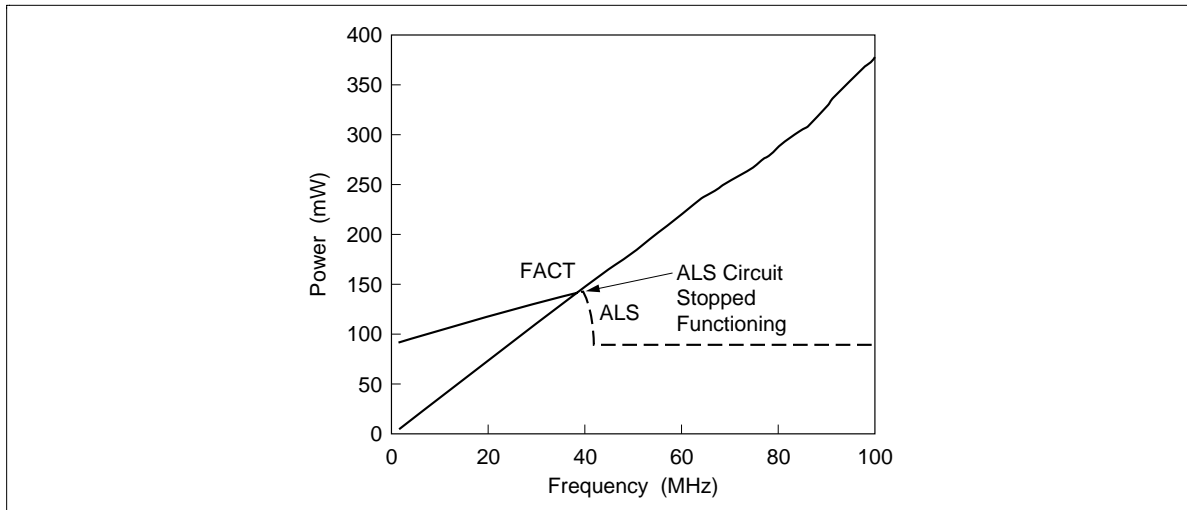
Figure 10 FACT vs ALS Circuit Power
