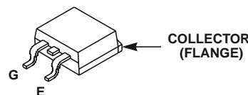
JEDEC TO-263AB
