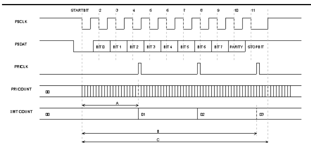
A: t_{PSTPRI} , B: t_{PSTREC} , C: t_{REC}
