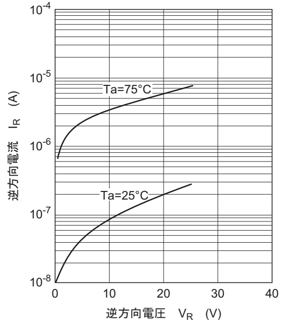
图2. 逆方向特性
