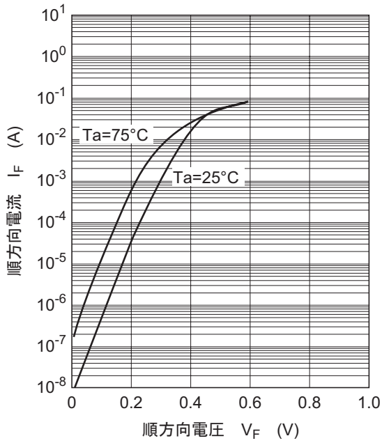
图1. 順方向特性
