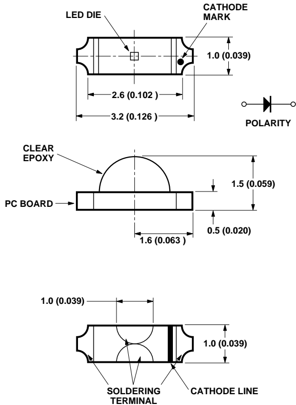
HSMB-C110
