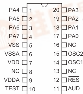
HT36A4 - 20 SOP-A
