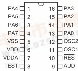
HT36A4 - 16 DIP-A
