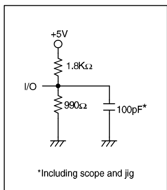
Output Load
