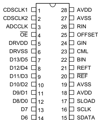
HT82V14 – 28 SOP/SOJ
