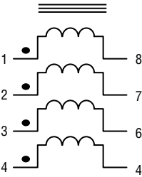
HT83-99654 & HT83-99655
