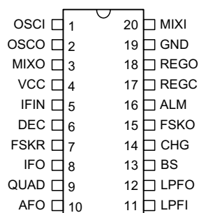
HT9011 - 20 SSOP
