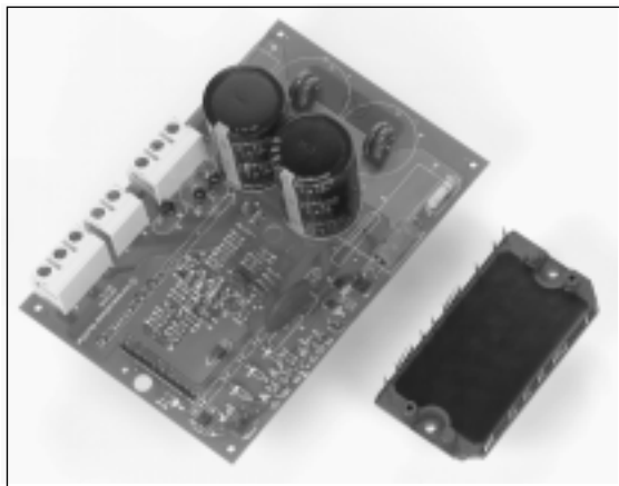
Figure 3. IRPT2059C POWIRTRAIN
