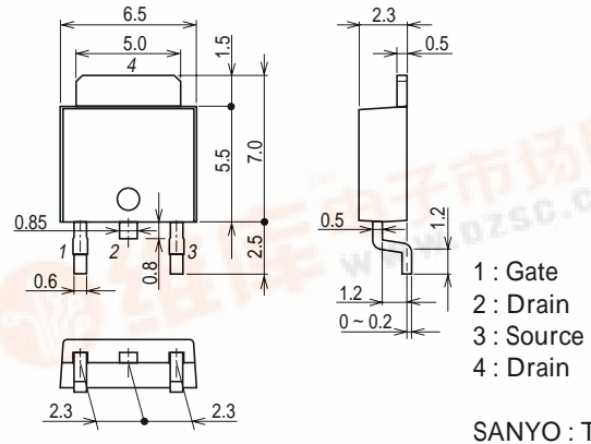
外形図 2092B
