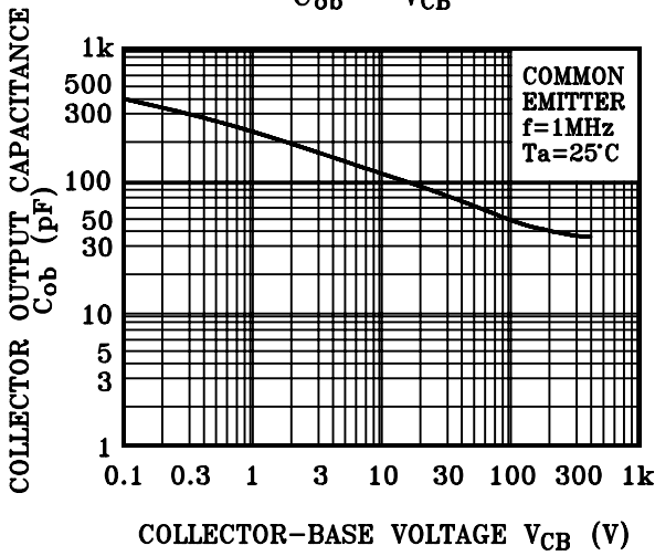
C_{ob} - V_{CB}
