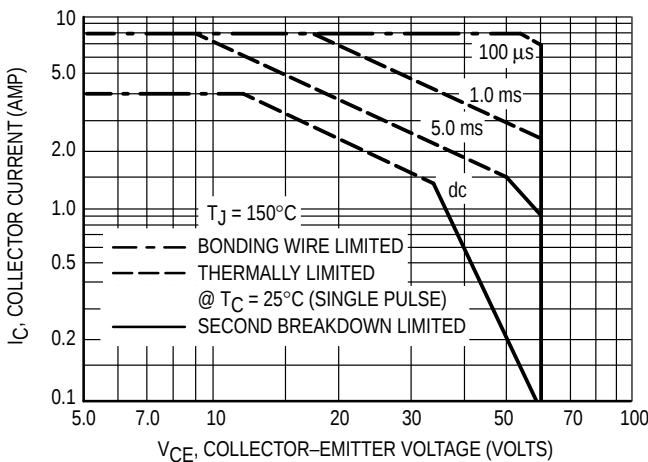
Figure 8. MJE700T
