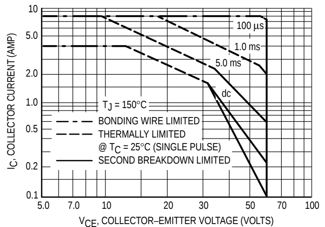
Figure 9. MJE800T
