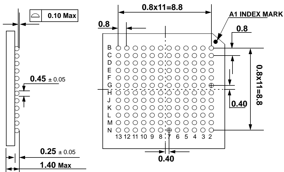
&lt;Bottom View&gt;
