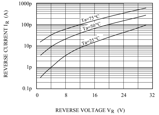
I_R - V_R
