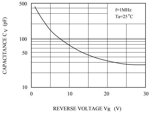
C_V - V_R
