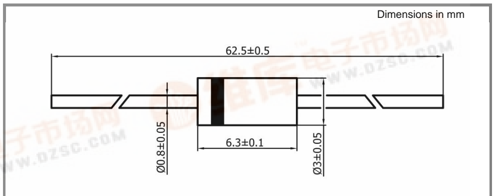
case: DO-15 / DO-204AC
