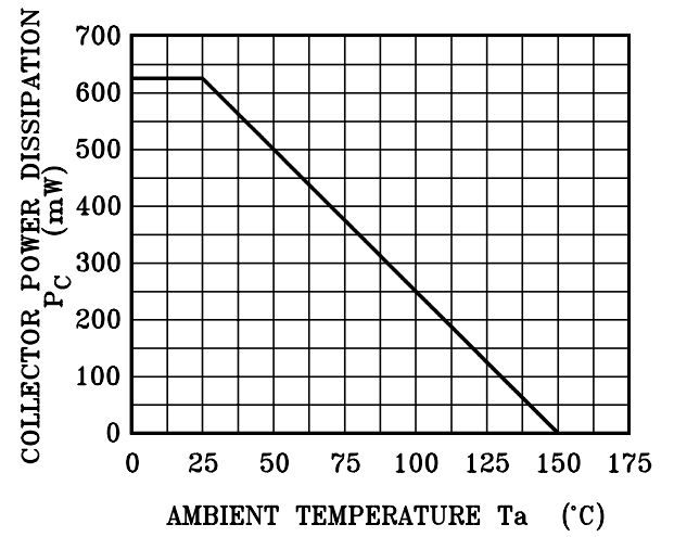
P_C - T_a
