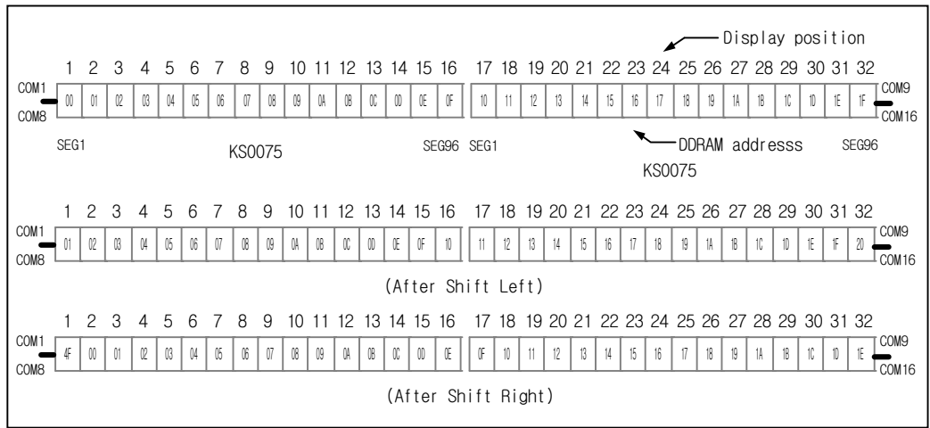
Fig-5. 1-line X 32ch. display
