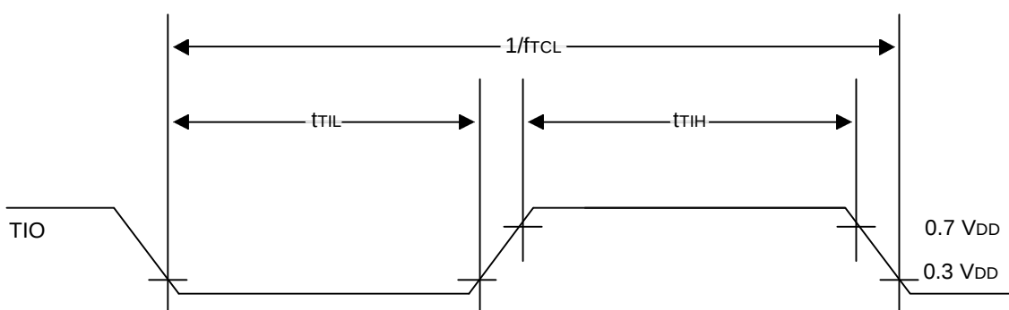
Figure 14-6. TIO Timing
