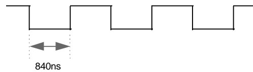
Fig. 2 NORMAL RESET
