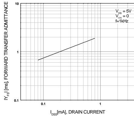
Figure 4. |Y_{FS}| - I_{DSS}
