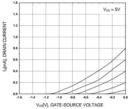
Figure 3. I_D - V_{GS}
