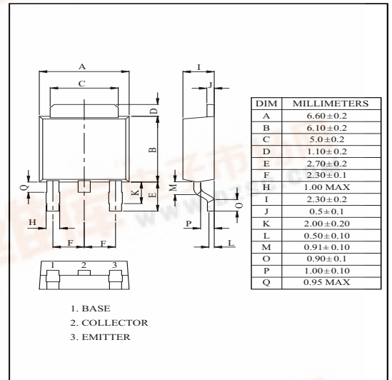
DPAK
