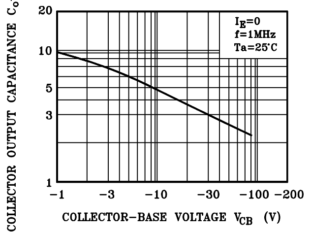
C_{ob} - V_{CB}
