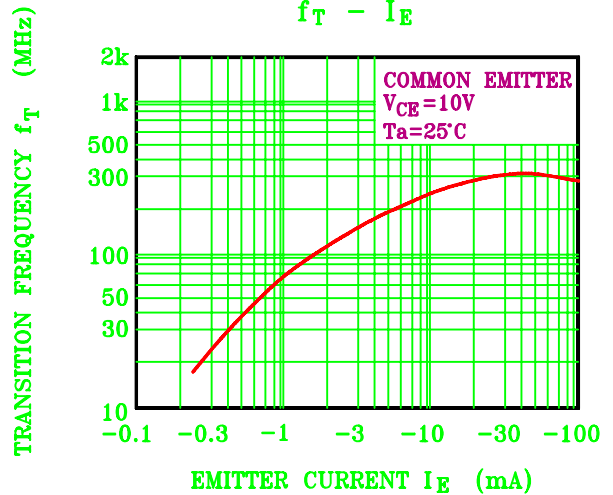
f_T - I_E
