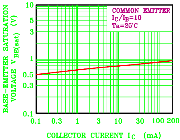
V_{BE(sat)} - I_C
