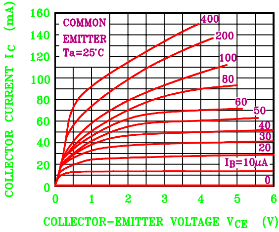
I_C - V_{CE}
