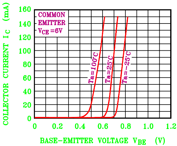
I_C - V_{BE}
