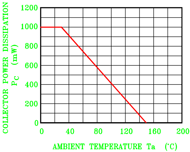
P_C - T_a
