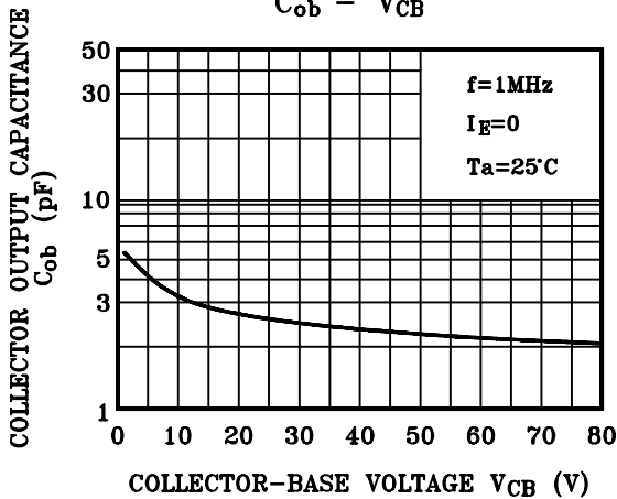
C_{ob} - V_{CB}
