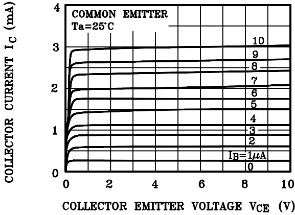
I_C - V_{CE}
