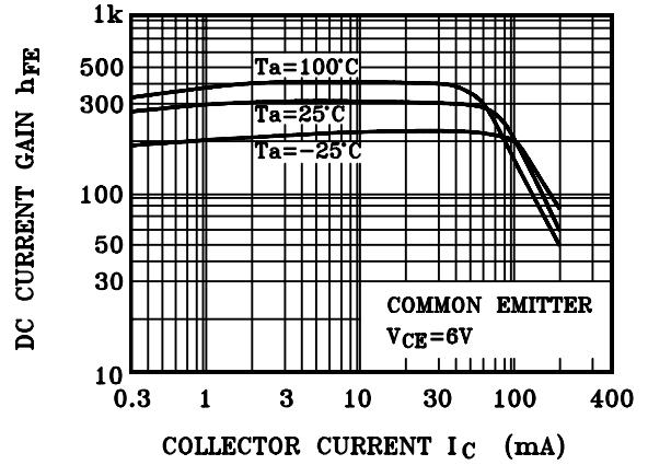
h_{FE} - I_C
