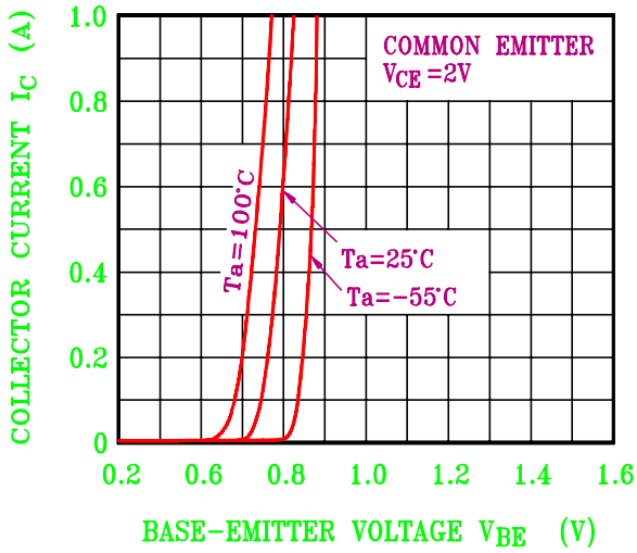
I_C - V_{BE}
