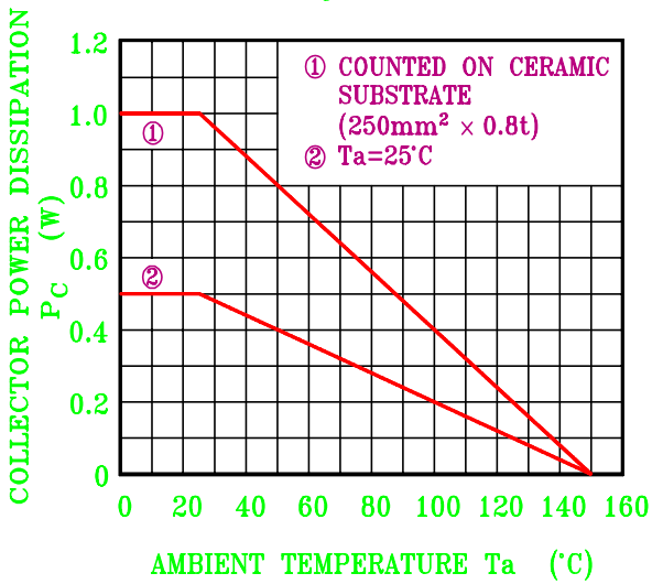
P_C - T_a
