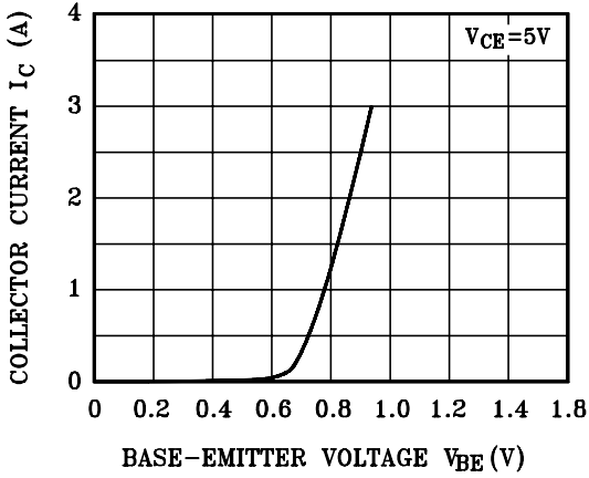
I_C - V_{BE}
