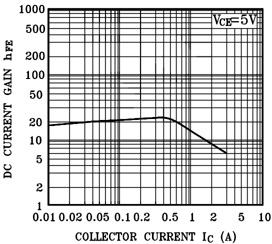
h_{FE} - I_C
