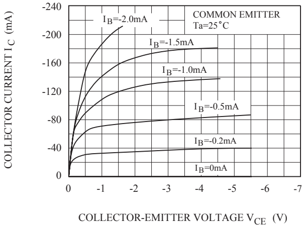
I_C - V_{CE}
