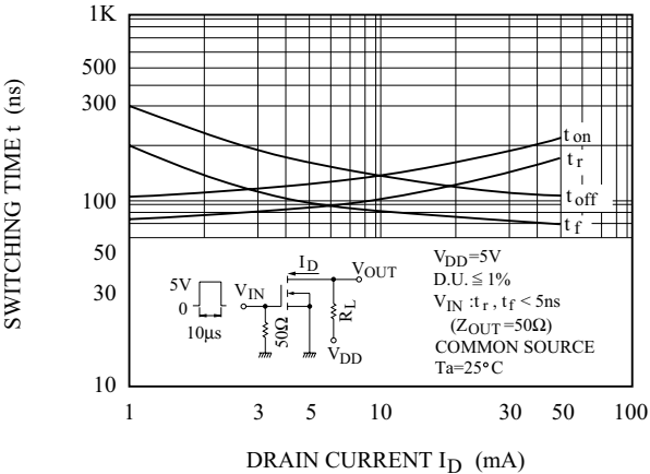
t - I_D
