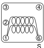
FM DET (DM6000DEAS-8407GLF)
