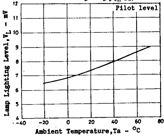
V_L - T_a (Fig 25)
