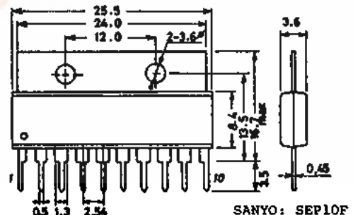
外形図 3018A-S10PIC (unit: mm)
