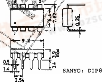
LA5521D 外形図 3001A-D8IC (unit: mm)
